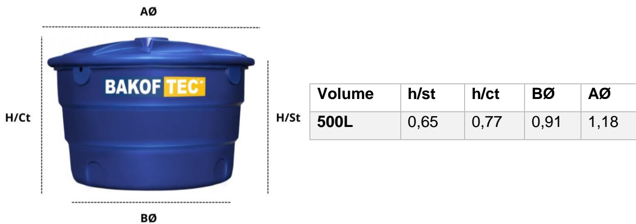
Figura 01. Desenho Reservatório 500L Bakof Tec*.
