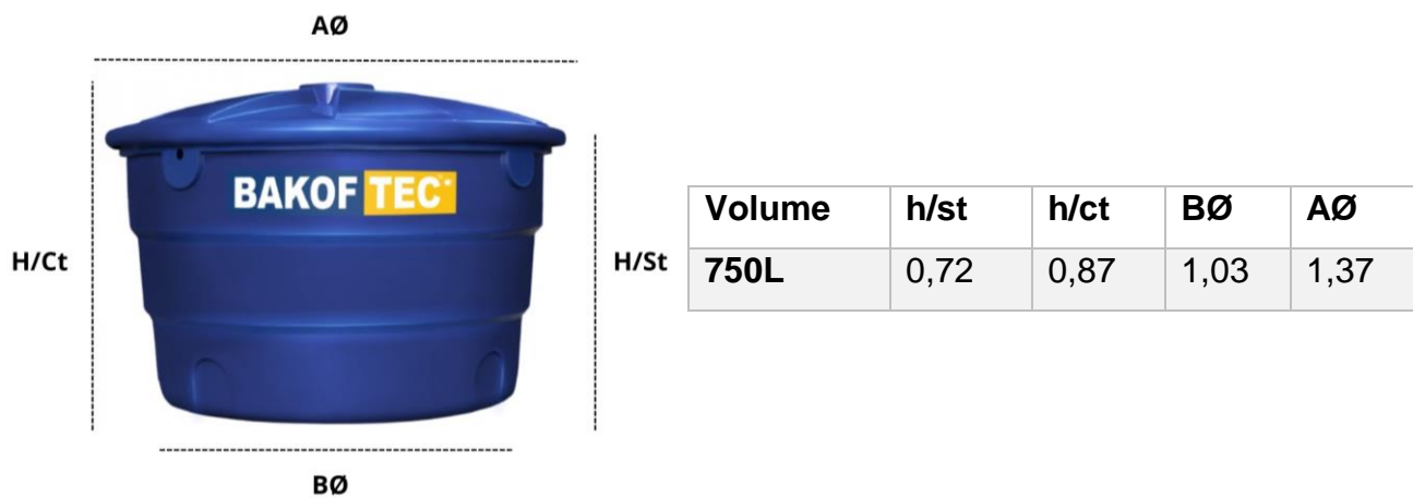
Figura 01. Desenho Reservatório 750L Bakof Tec*.
