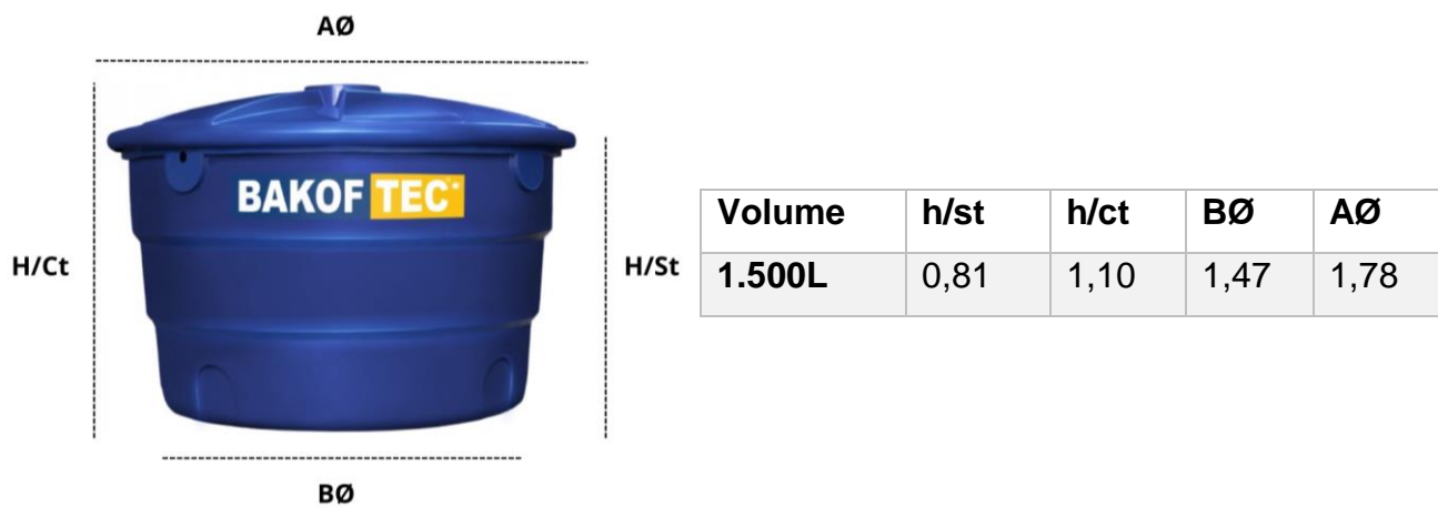
Figura 01. Desenho Reservatório 1.500L Bakof Tec*.
