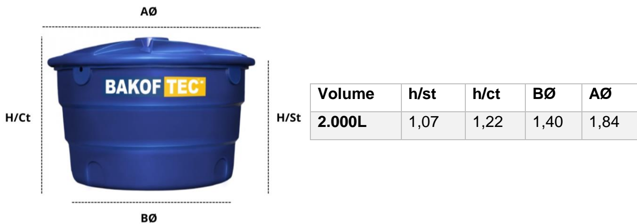
Figura 01. Desenho Reservatório 2.000L Bakof Tec*.
