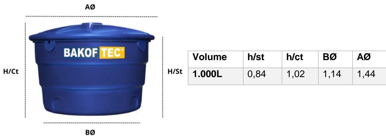
Figura 01. Desenho Reservatório 1.000L Bakof Tec*.
