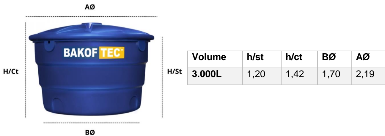
Figura 01. Desenho Reservatório 3.000L Bakof Tec*.
