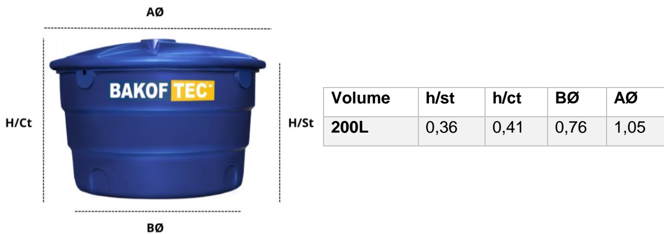
Figura 01. Desenho Reservatório 200L Bakof Tec*.
