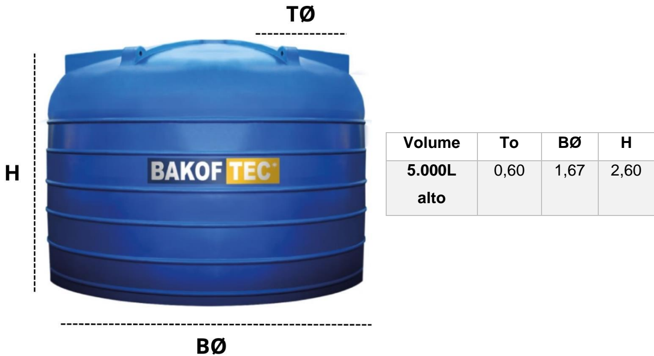
Figura 01. Desenho Tanque 5.000L alto Bakof Tec*.
