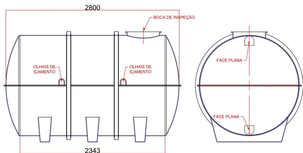
Figura 01: Esquema com as medidas básicas – Tanque Cilíndrico Horizontal.
