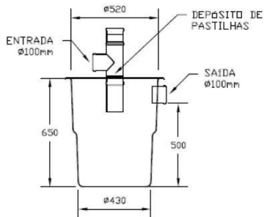
Figura 1. Desenho ilustrativo Clorador 100 L.
